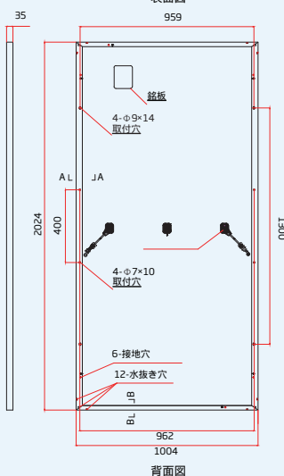
背面図
